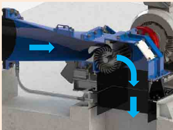
水車内部構造図 (イメージ)
