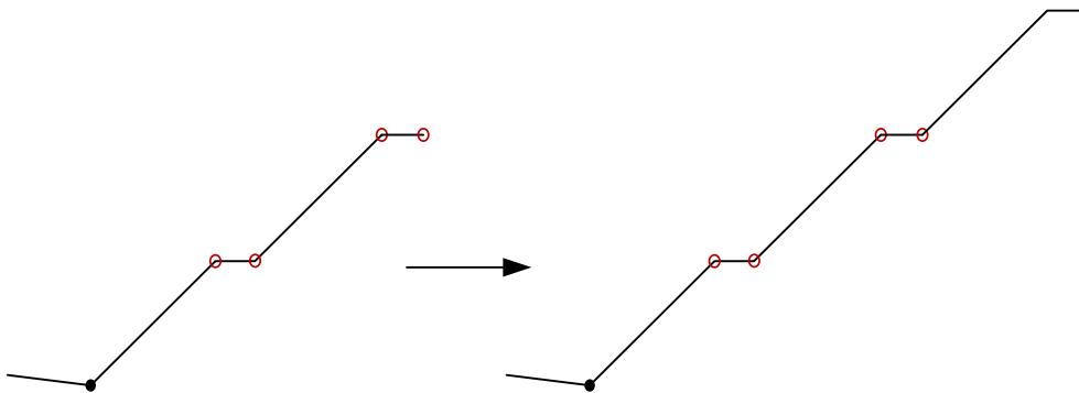
図 4-16 法面と小段の定義方法（小段で終わる場合）
