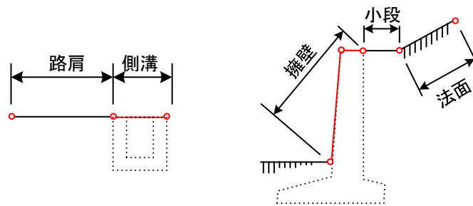
図 4-22 構造物『表面』の作成方法（左：側溝 右：擁壁）
