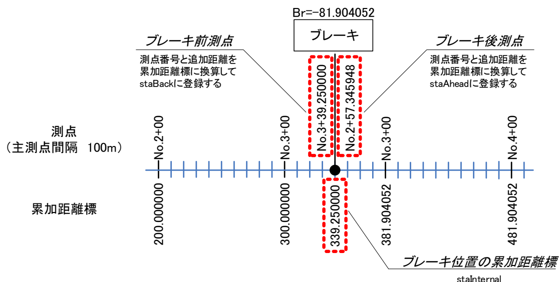
図 4-5 ブレーキ前後の測点番号とブレーキ位置の累加距離標の関係
