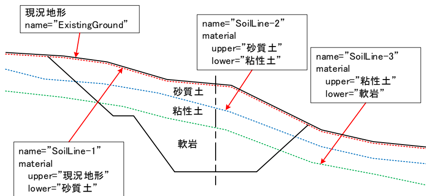
図 4-30 地形線を用いた地層表現例 (1)
