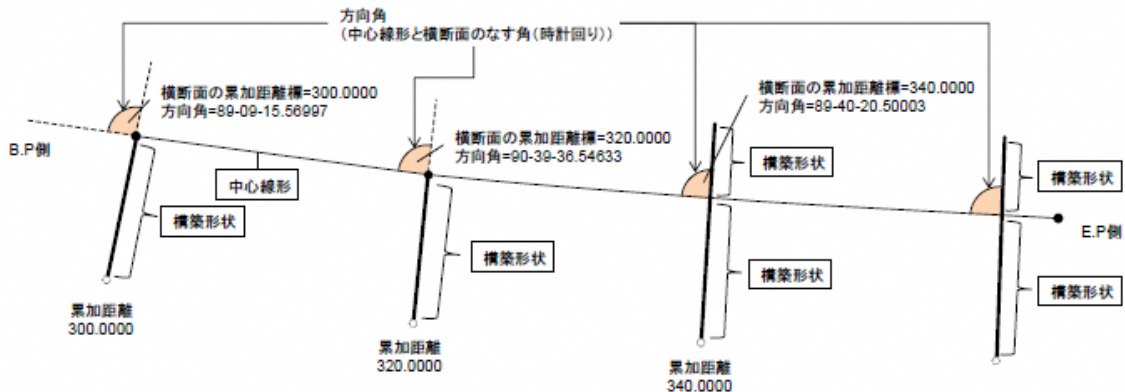
図 4-11 方向角の解説
