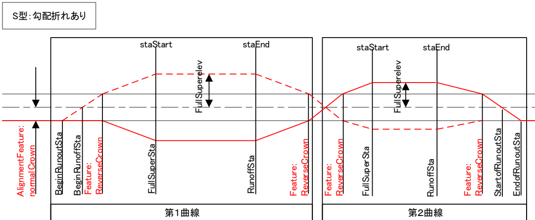
図 4-8 片勾配すりつけの例 (S型)
