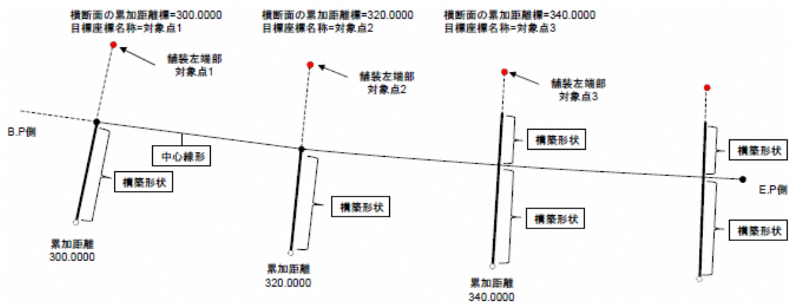
図 4-12 目標座標名称の解説
