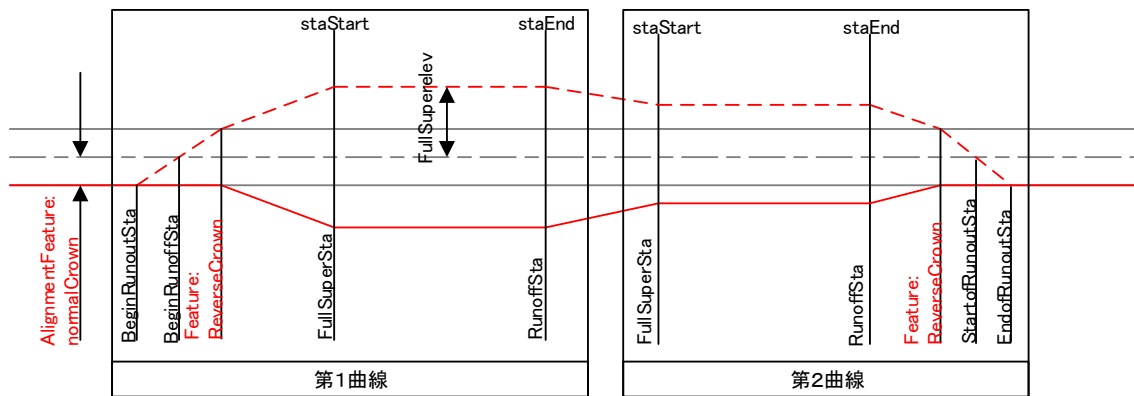
図 4-9 片勾配すりつけの例 (卵型)
