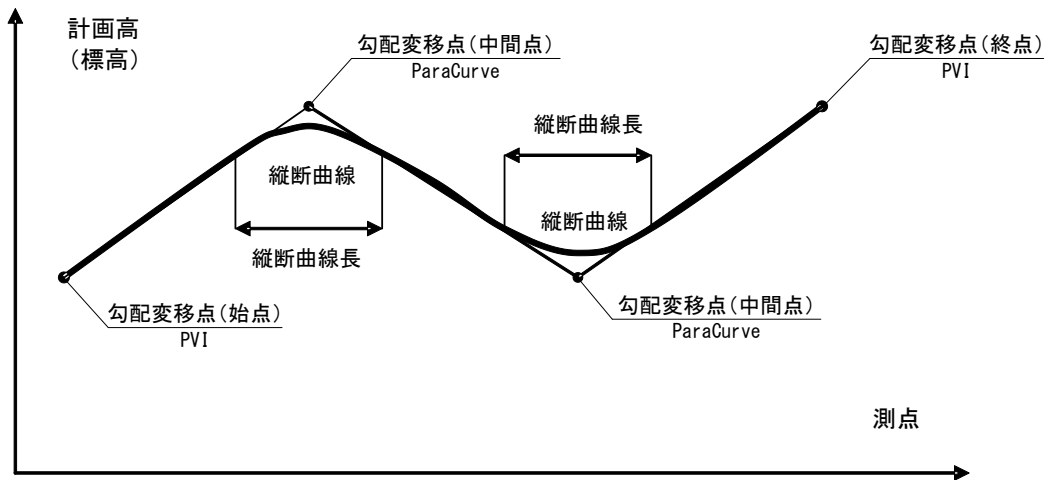
図 4-10 縦断線形と勾配変移点の関係
