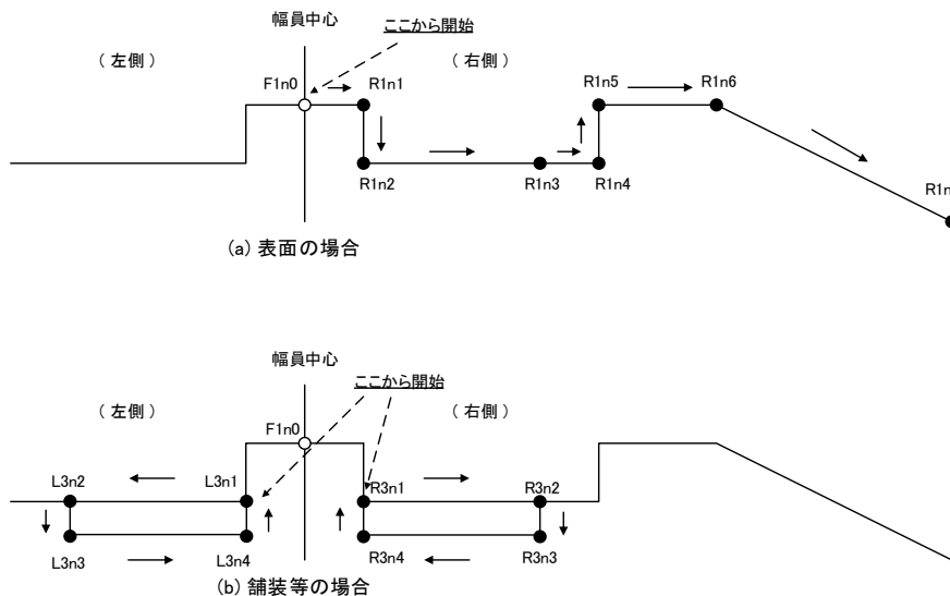
図 4-17 構成点を記載する順序 (コード番号は例)
