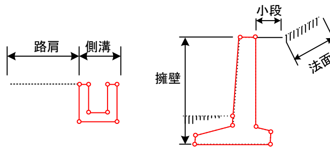
図 4-23 構造物『外周』の作成方法（左：側溝 右：擁壁）
