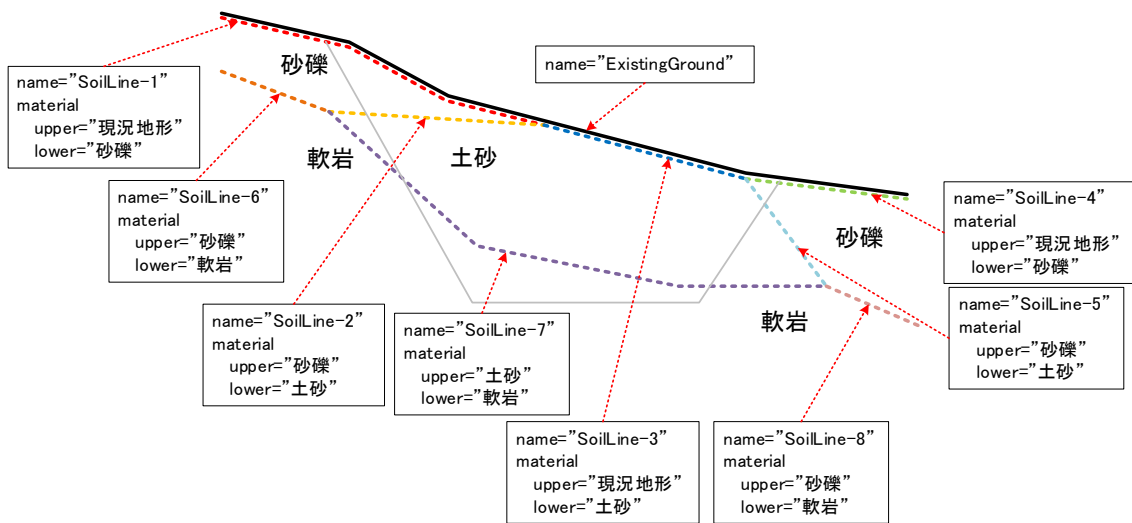
図 4-31 地形線を用いた地層線の例（2）
