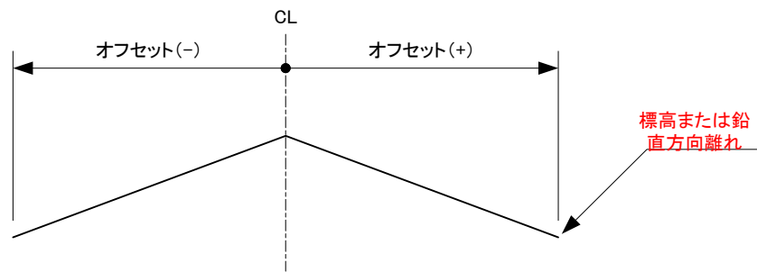
図 4-19 オフセットと標高または鉛直方向離れ (OffsetElevation)
