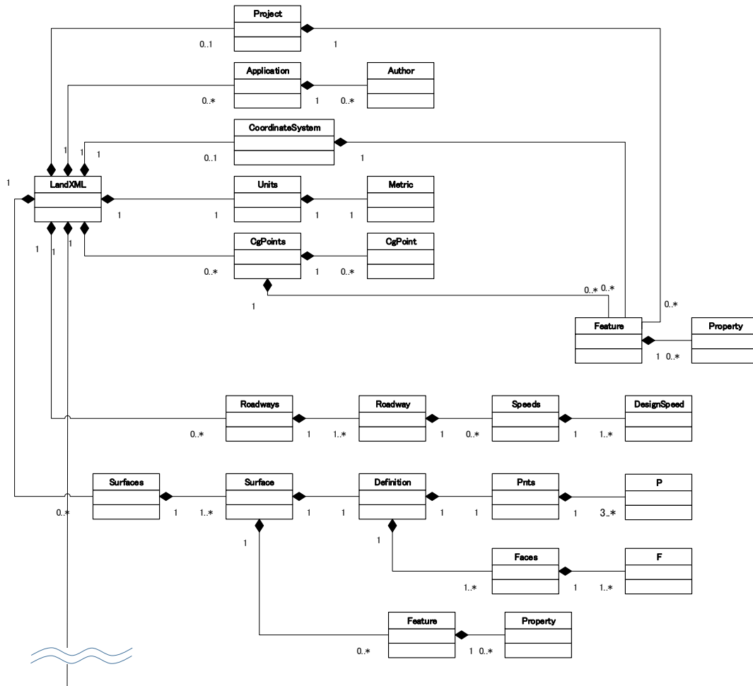
図 4-34 UML クラス図による表現
