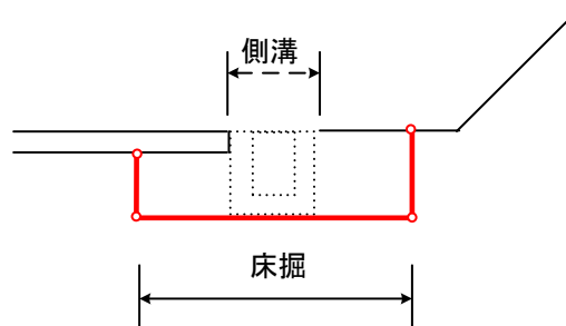
図 4-24 床掘の作成方法
