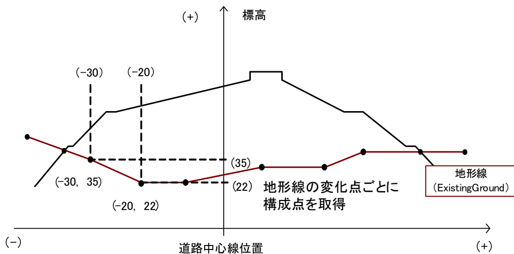
図 4-29 地形情報と 2 次元座標リストの定義方法
