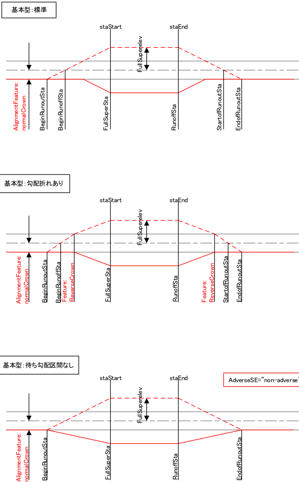
図 4-7 片勾配すりつけの例 (基本型)
