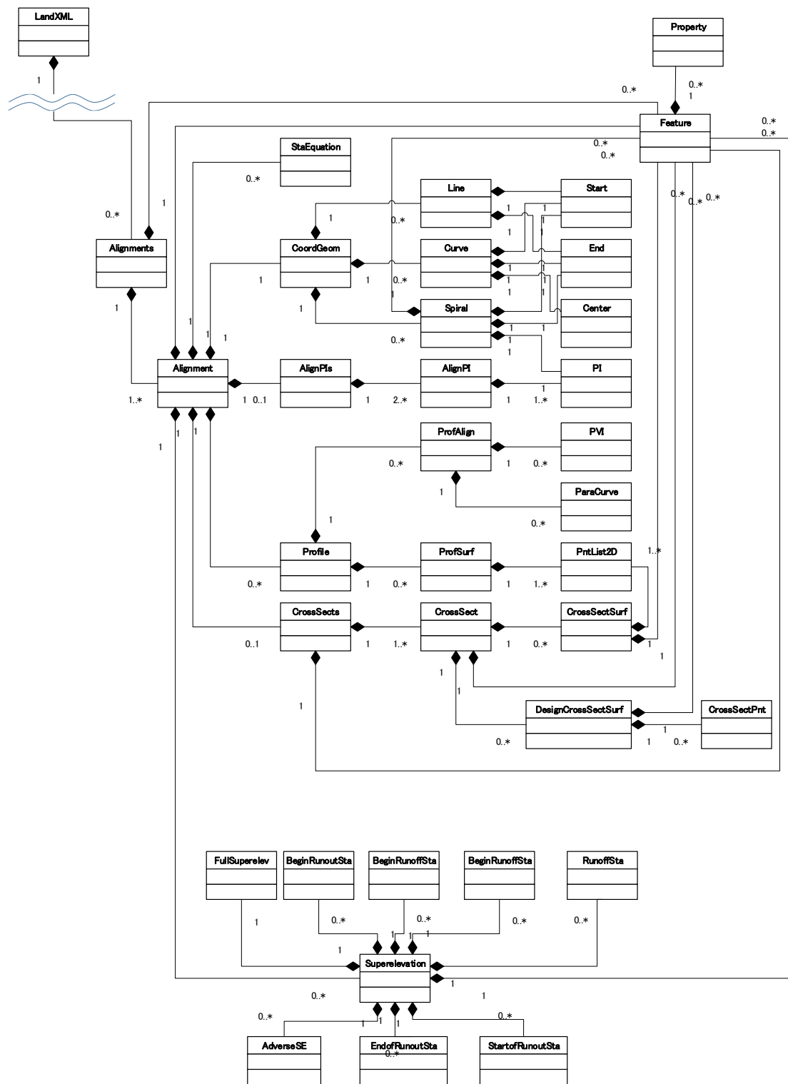
図 4-35 UML クラス図による表現 (Alignments 配下)
