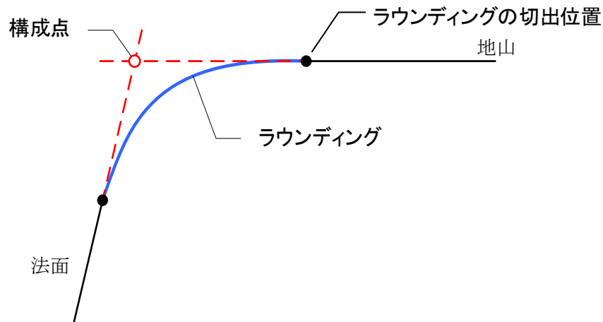
図 4-13 ラウンディングの定義方法
