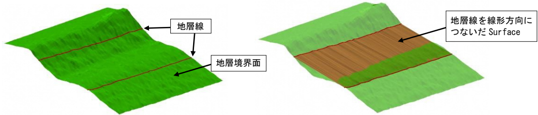
図 4-32 地層線を線形方向につないだサーフェスの例
