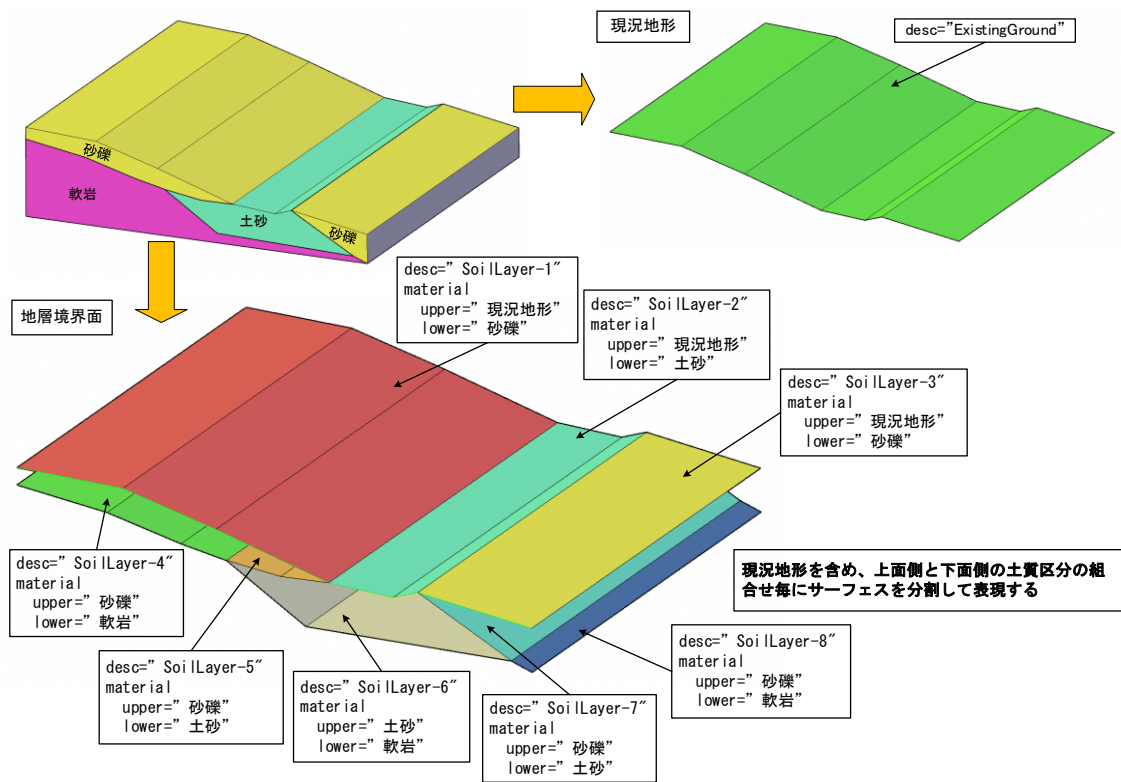
図 4-33 サーフェスを用いた地層表現例
