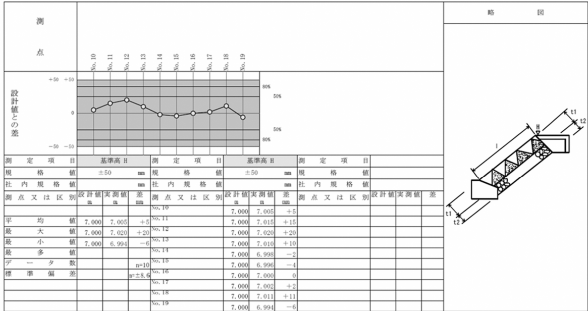
図-3 作成帳票例 (出来形管理図表)
