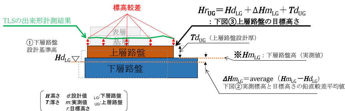
図2-7 標高較差の算出ロジックのイメージ (例:アスファルト舗装)
