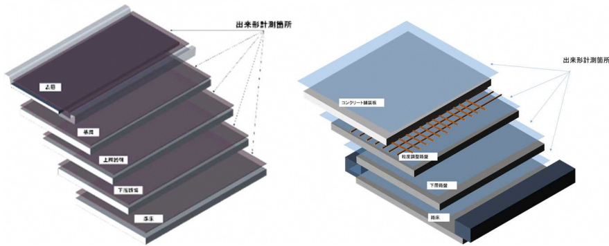
(コンクリート舗装)
