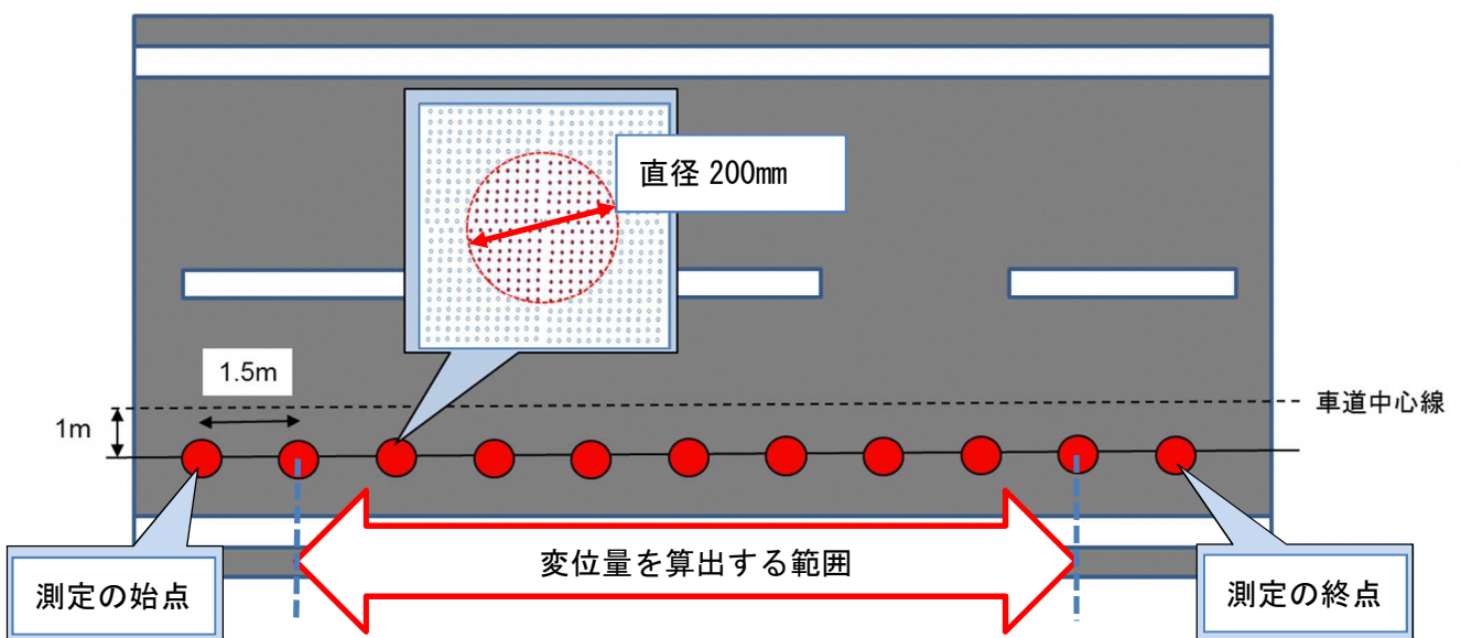
参考資料図 5-1 計測点群データによる平坦性算出のイメージ
