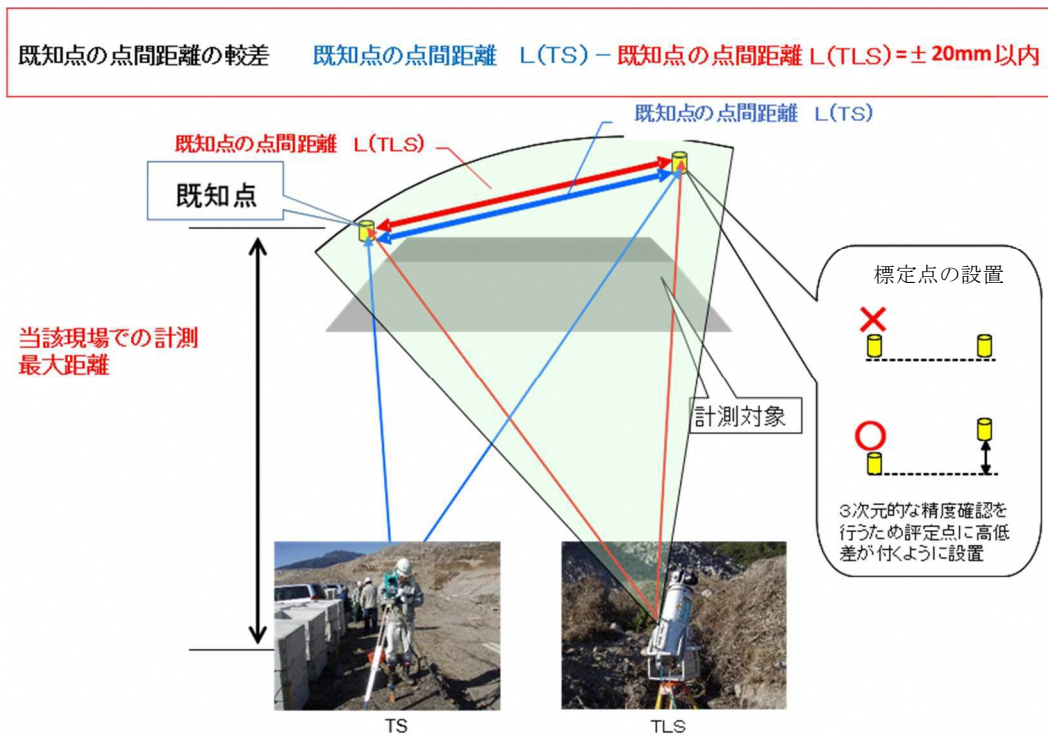
参考資料図 4-2 精度確認試験の配置イメージ図
