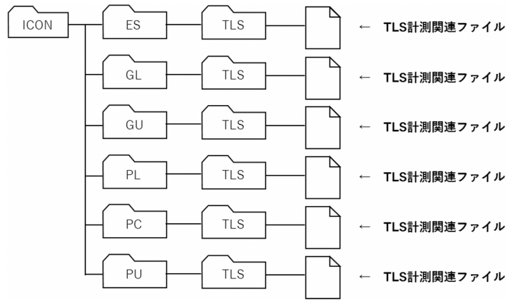
図5-9 フォルダ構成例（現況地形（路床）の起工測量、下層路盤・上層路盤・基層・中間層・表層を計測した場合）
