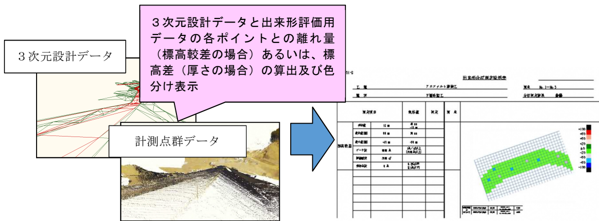
図5-1 出来形管理図表 作成の流れ
