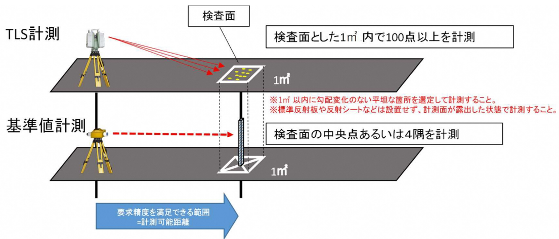
参考資料図 4-1 精度確認試験の配置イメージ図
