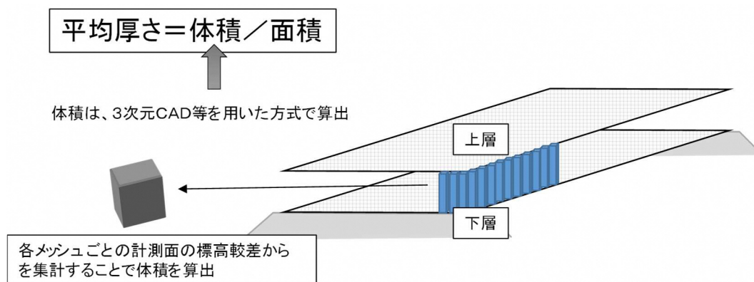
図5-5 平均厚さの数量算出イメージ（点高法による）
