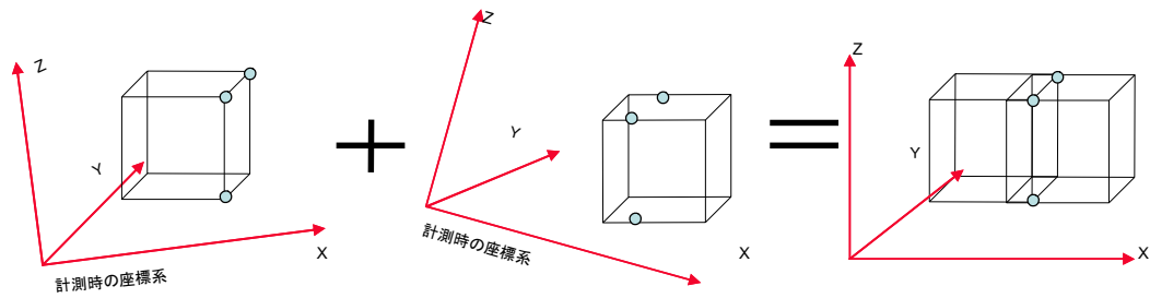
図 2-5 複数のスキャンに含まれる標定点を基準に合成する方法
