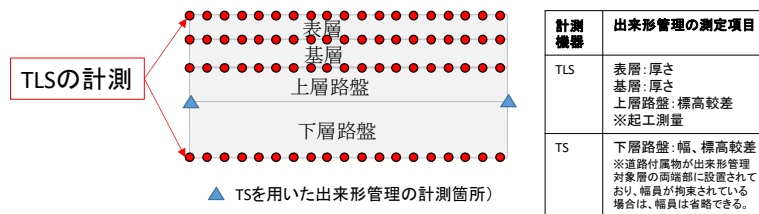
図4-4 TLSとTSを組み合わせた出来形管理例(例:アスファルト舗装)
