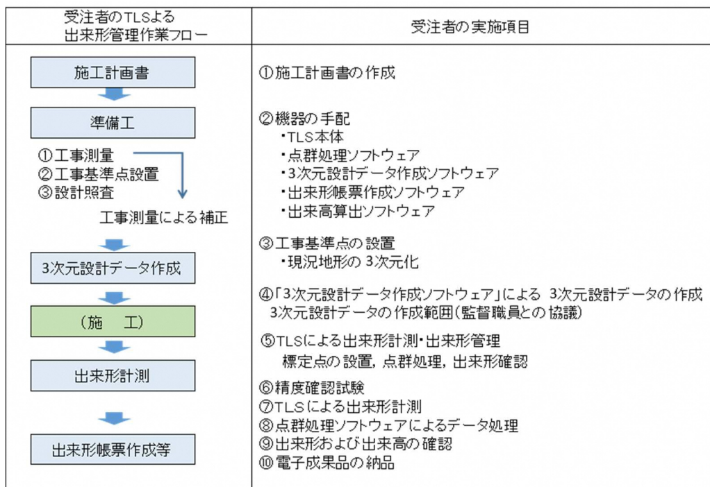
図 1 - 1 出来形管理の主な手順
