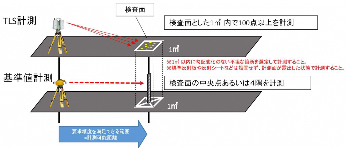
参考資料図 4-3 T L S の精度確認方法
