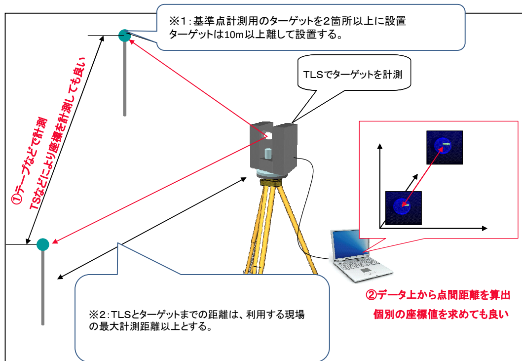
参考資料図 4-4 TLSと既知点の設置
