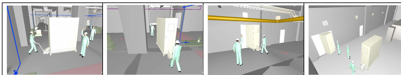
図 39 施工手順の検討において BIM/CIM モデルを利用した例 (LOd : 30 相当)
