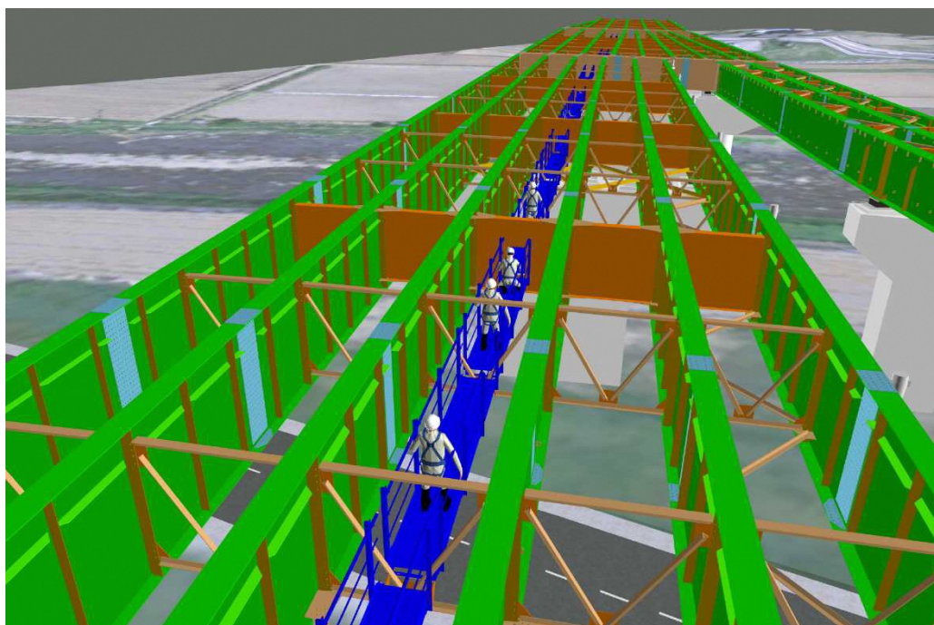
図 29 点検路の導線・狭隘箇所確認
