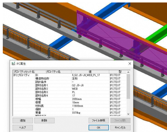
図 24 属性情報の目視による確認イメージ
