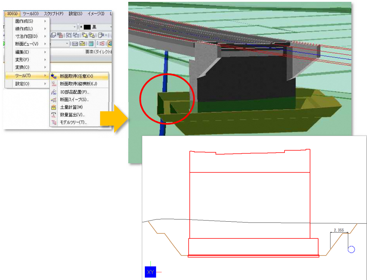
図 9 3DA 面図による埋設管と基礎工の離隔確認イメージ
