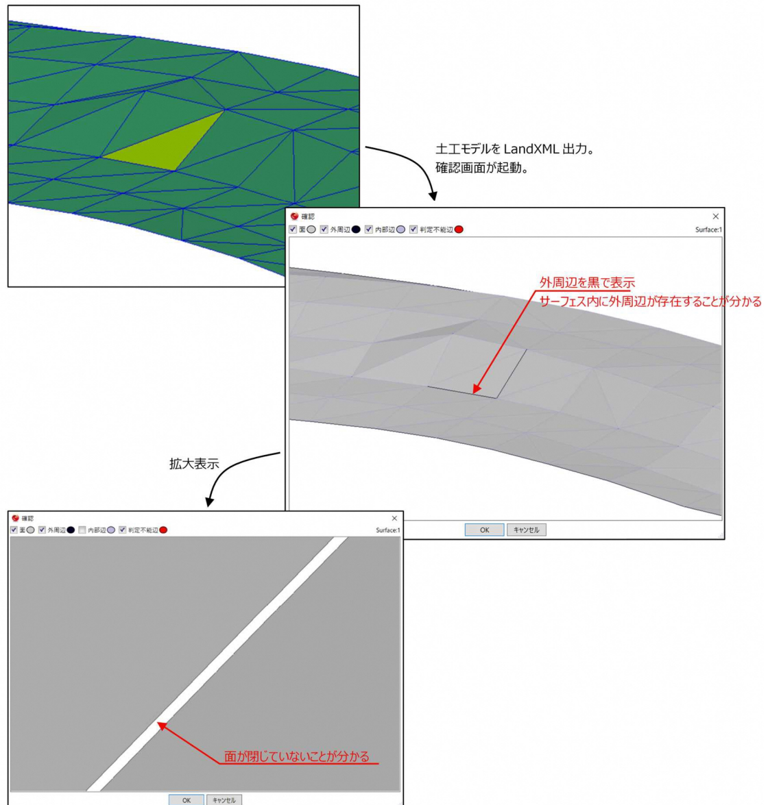
図 20 非接続エッジ検出機能によるサーフェス接続の確認イメージ（土工）
