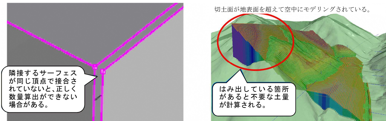
図 17 BIM/CIM モデル不備の例
