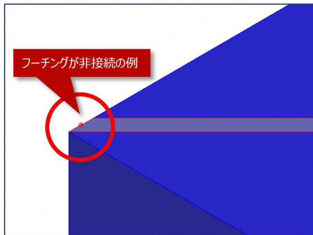
図 19 非接続エッジ検出機能によるサーフェス接続の確認イメージ（構造物）
