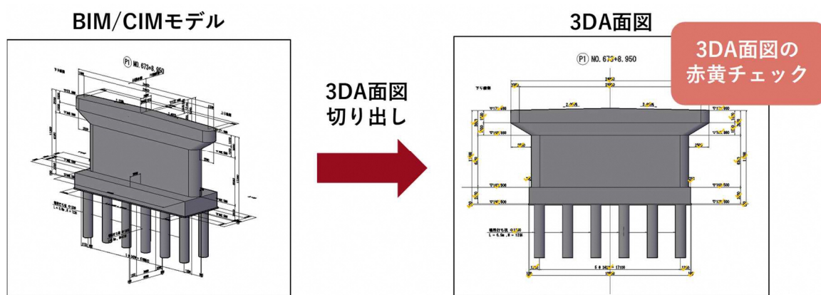
図 16 3DA 面図の赤黄チェック
