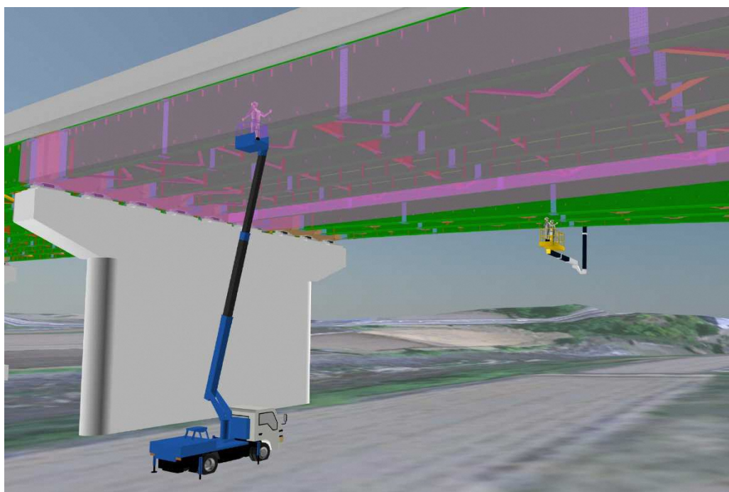
図 28 点検シミュレーションによる点検範囲確認
