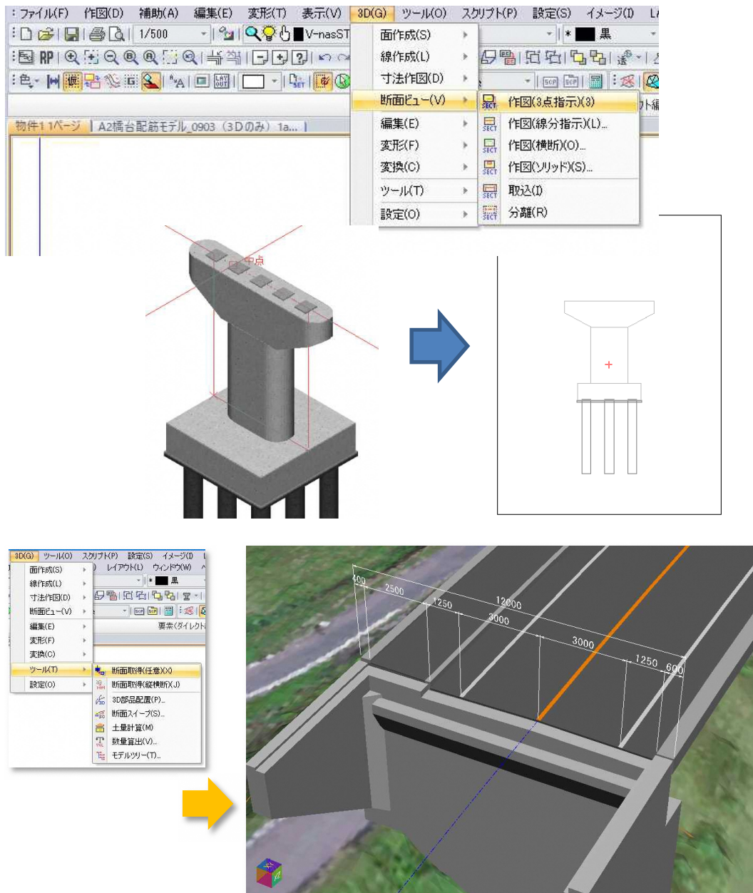
図 18 アノテーション機能にて作成した寸法による確認イメージ
