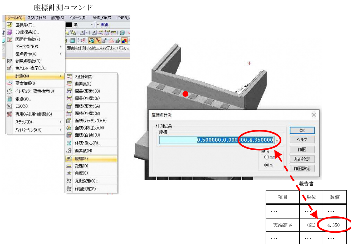
図 5 3DA モデルの座標と設計値の比較イメージ
