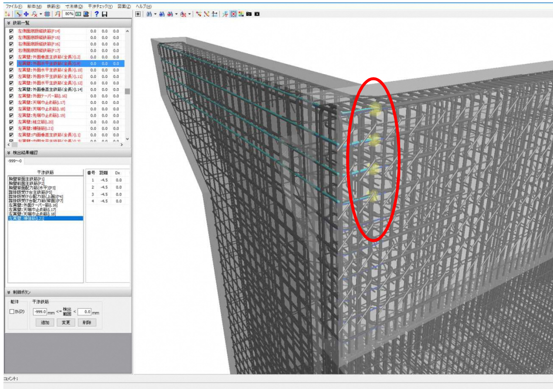
図 11 3D 配筋図による干渉箇所の確認イメージ
