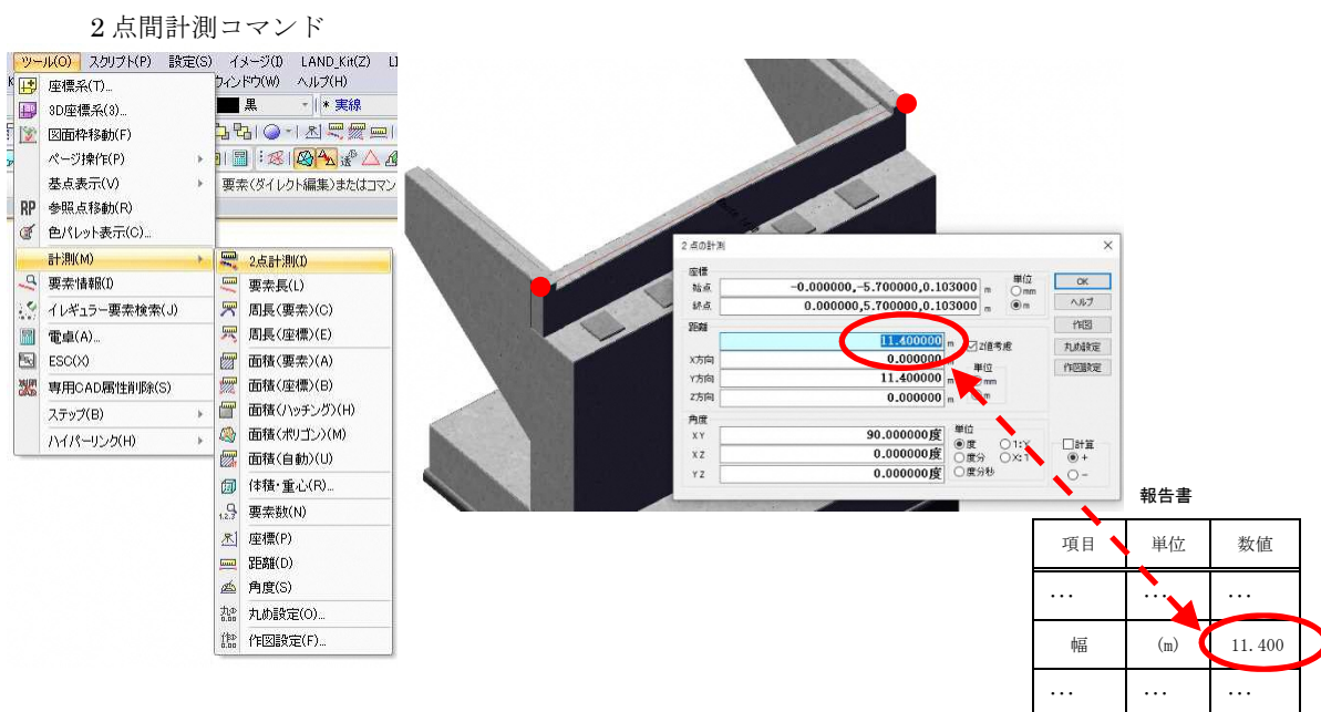
図 3 3DA モデルの計測値と設計値の比較イメージ
