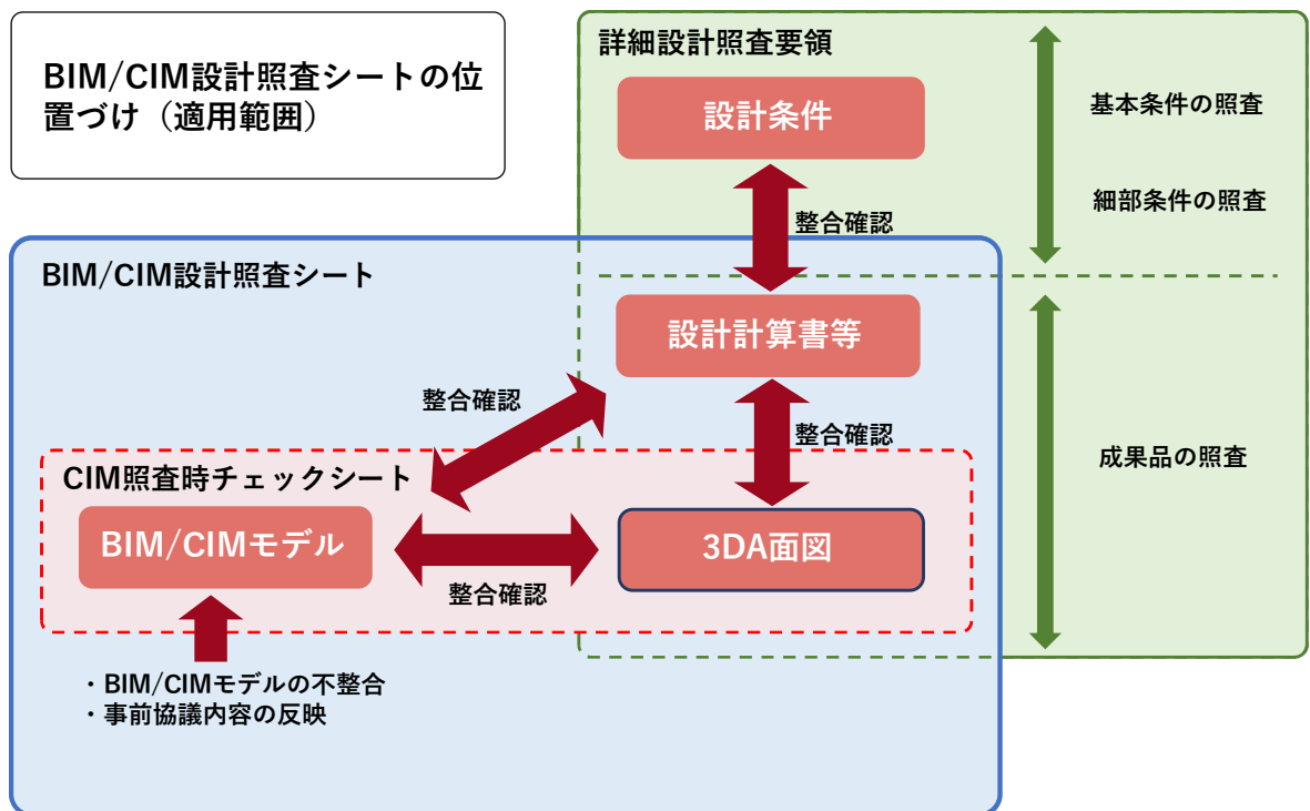
図 2 BIM/CIM 設計照査シートの適用範囲
