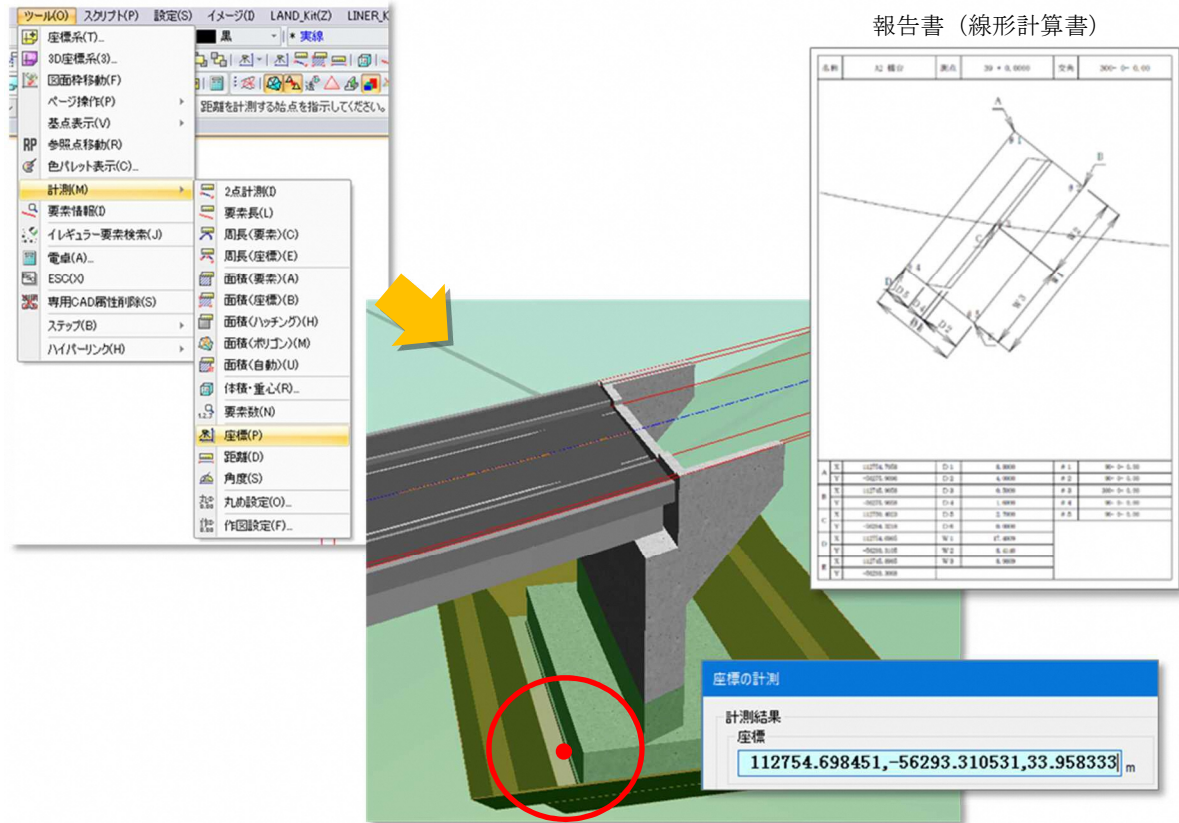
図 7 座標計測値と報告書との比較イメージ
