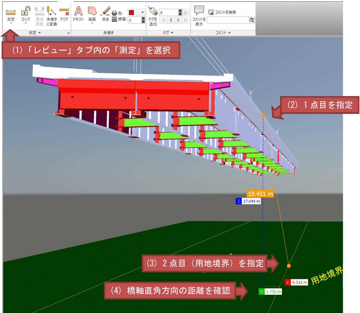
図 14 用地境界との離隔距離確認イメージ
