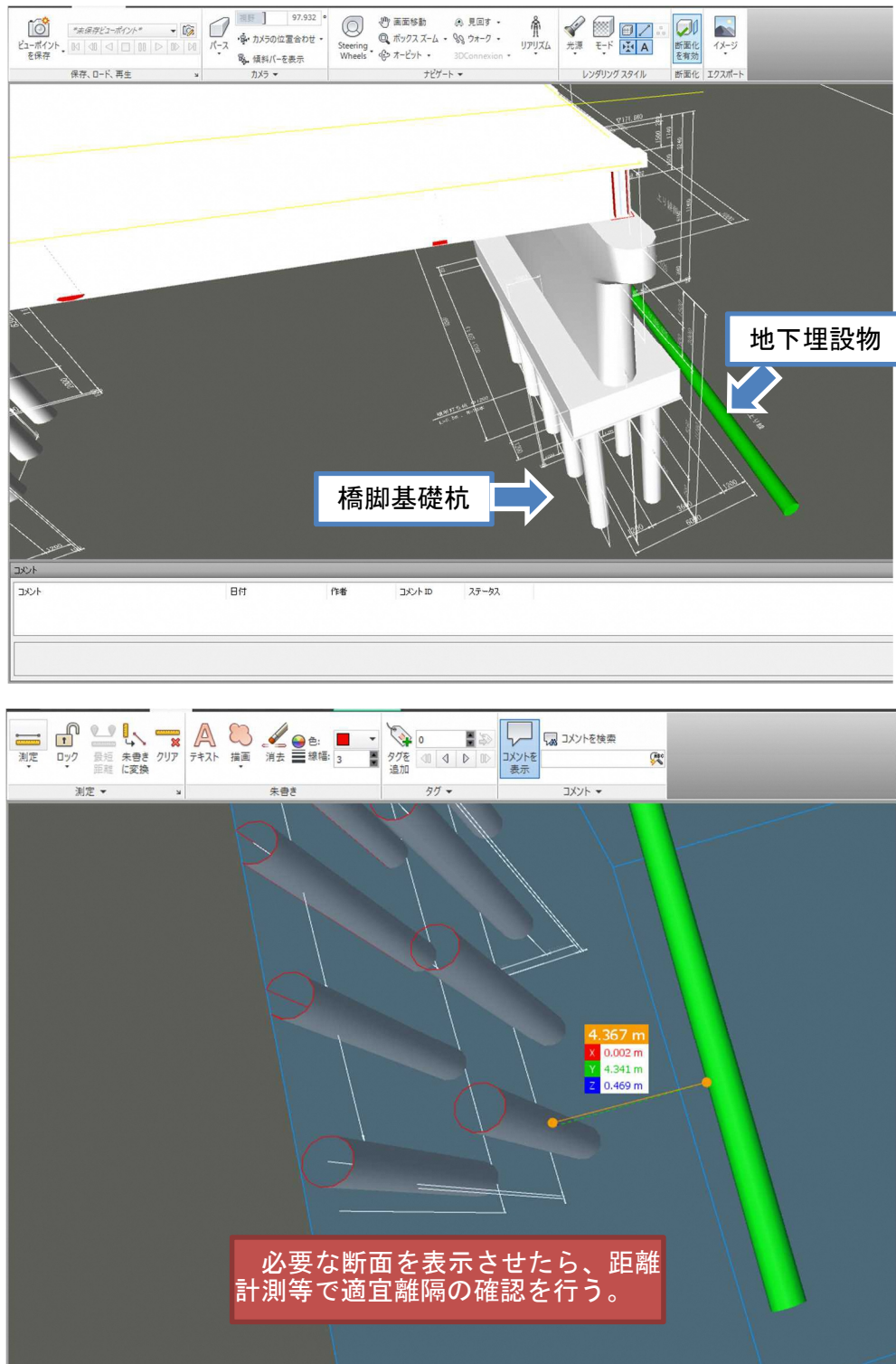
図 8 BIM/CIM モデルによる杭と地下埋設物の離隔距離確認イメージ
