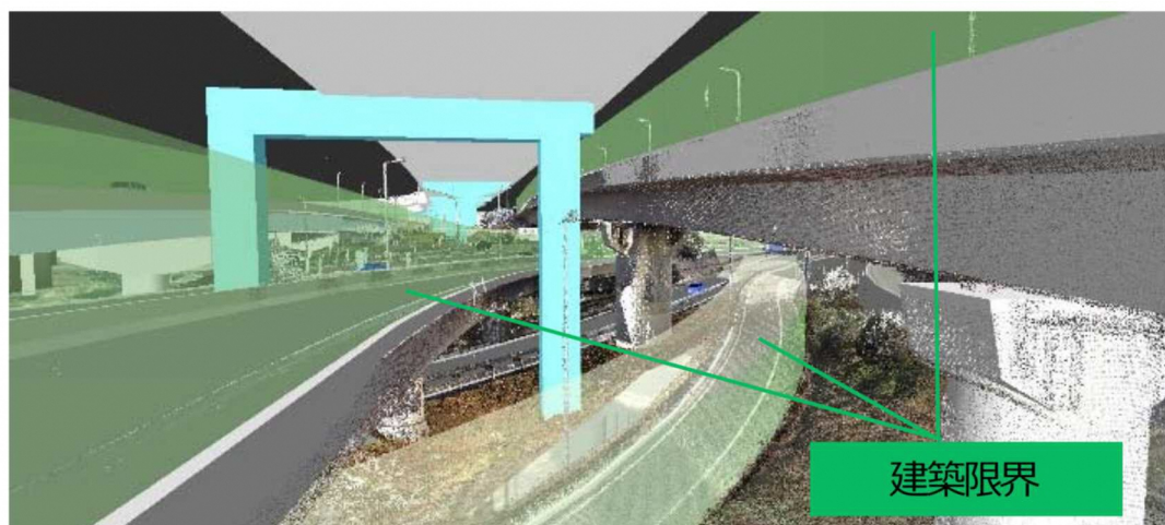
図 27 BIM/CIMモデルによる建築限界の確認
