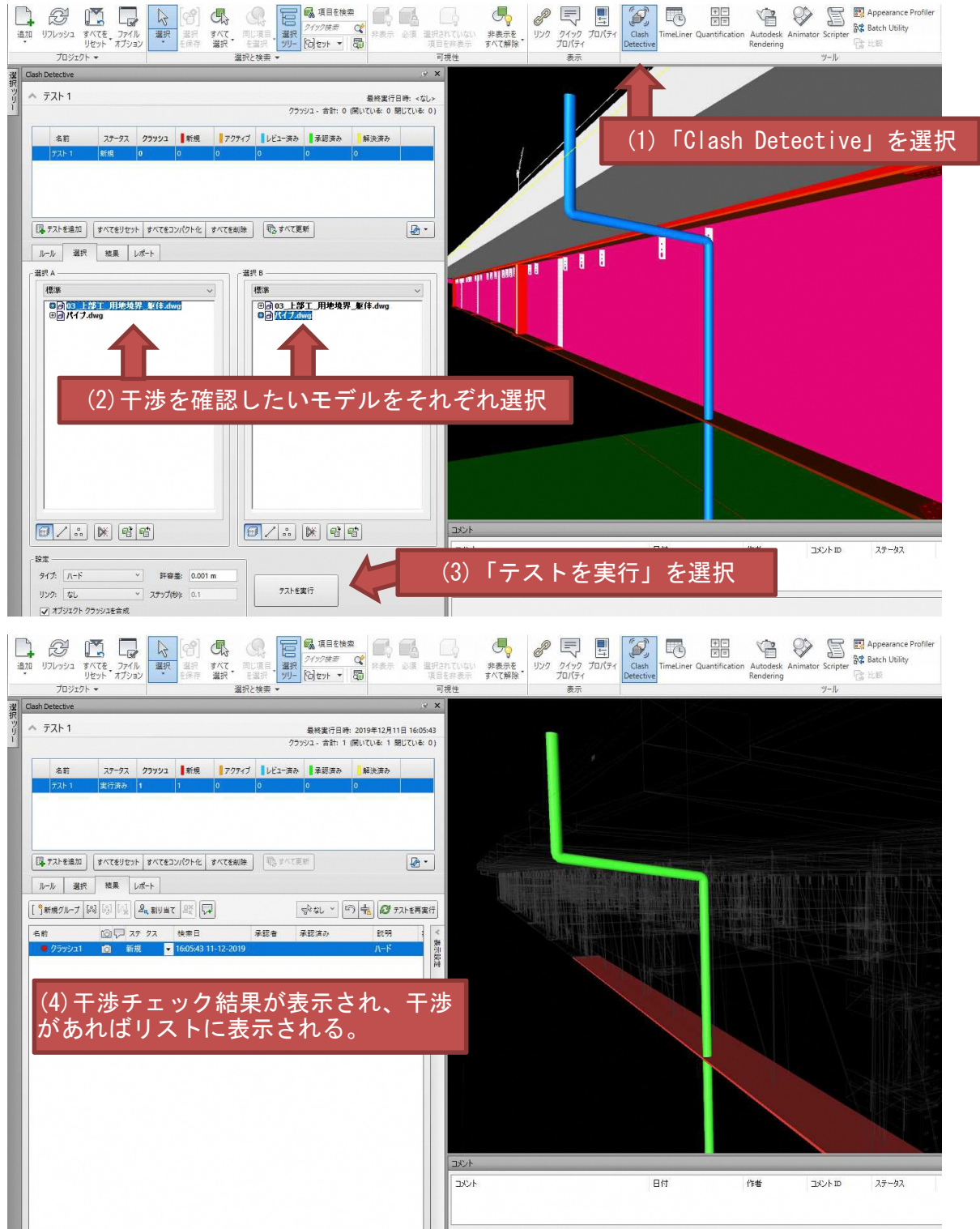
図 10 縦桁と排水管の干渉有無の確認イメージ
