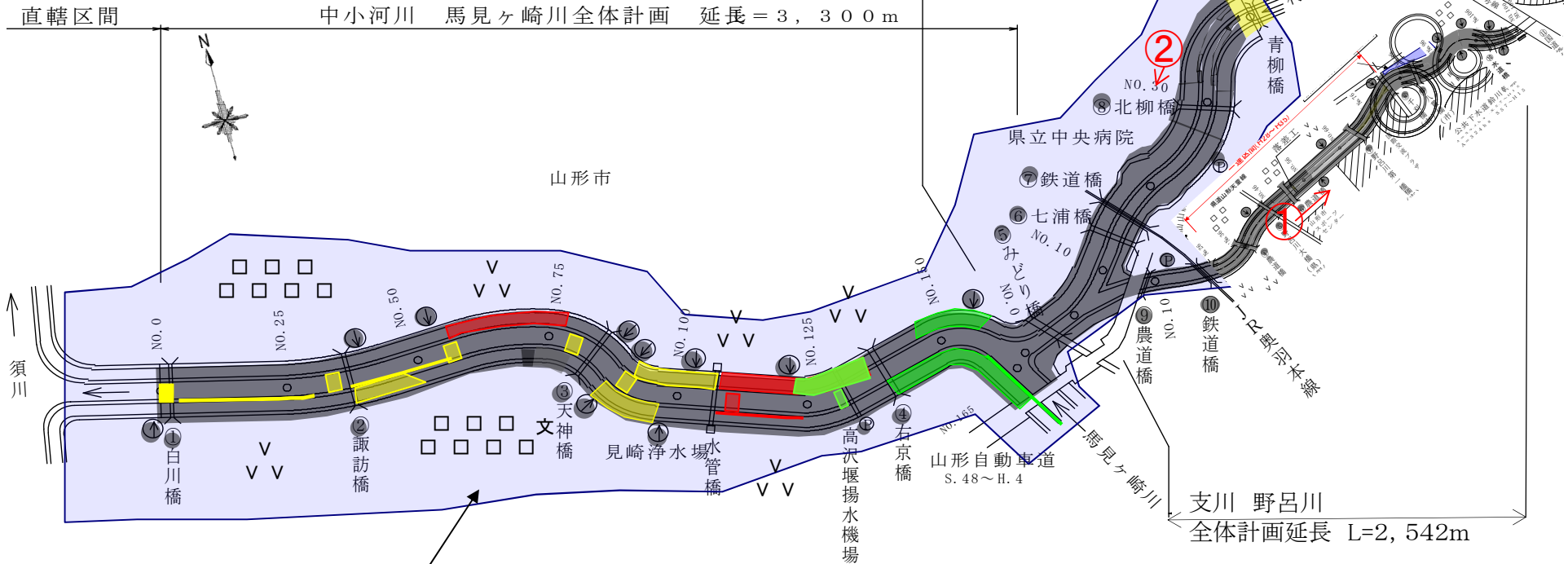
村山高瀬川 北柳橋より下流を望む 平成19年9月7日台風9号 出水状況
