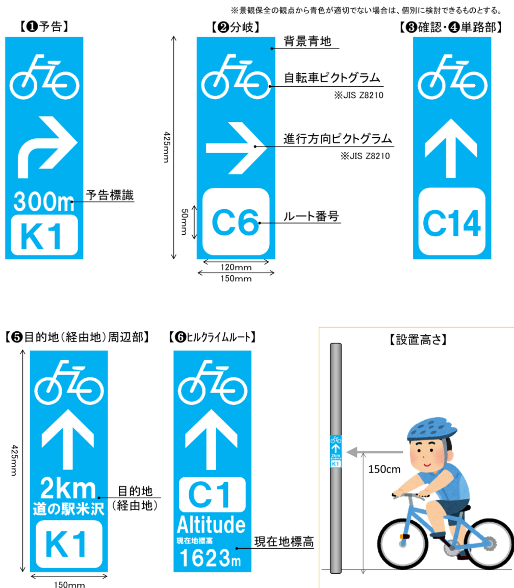
図 4-2 案内看板の標準仕様
