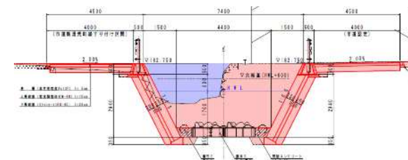
計画断面図
