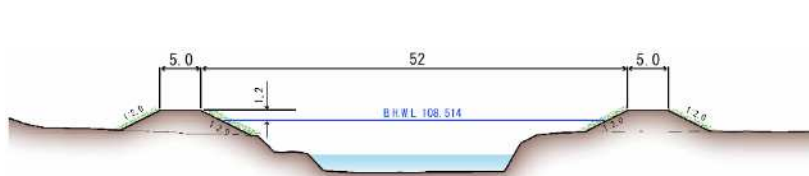
河川整備計画断面図
