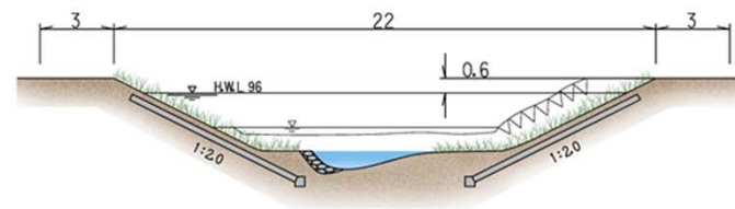
河川整備計画断面図
