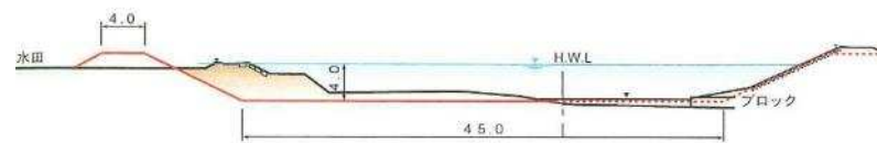
河川整備計画断面図 (最上川合流点から上流29.0km)
