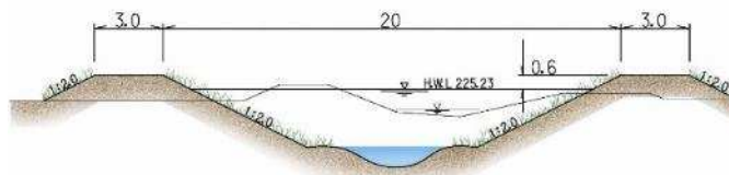
河川整備計画断面図（最上川合流点から上流8.5km）
