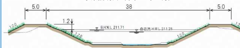
河川整備計画断面図 (最上川合流点から上流2.8km)
