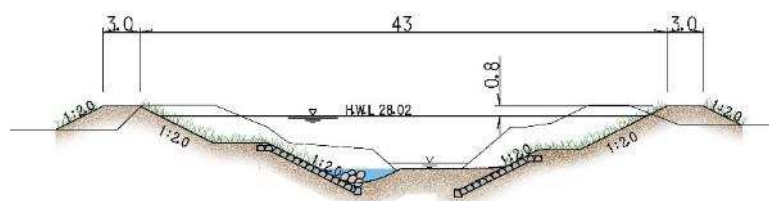
河川整備計画断面図 (相沢川合流点から上流1.0km)
