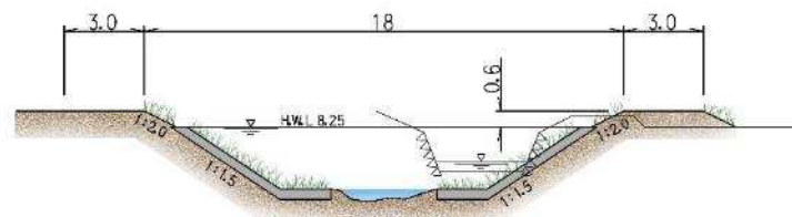
河川整備計画断面図 (京田川合流点から上流0.2km)
