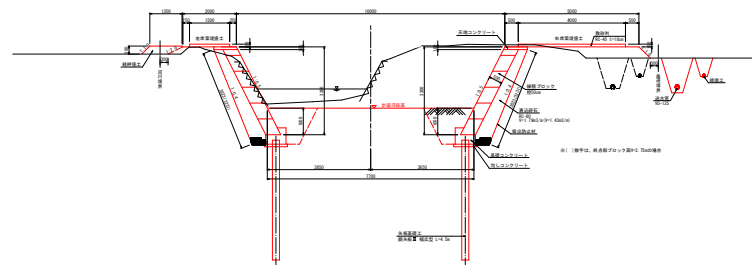
計画断面図
