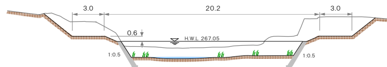
河川整備計画断面図 (置賜白川合流点から上流0.8km)
